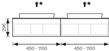
PLI02 2 Ladenelemente (Siphon-Laden)*
