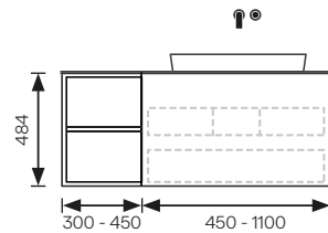
PLA06 1 Offenes Element 1 Ladenelement (Standard-Lade und Siphon-Innenlade)*
