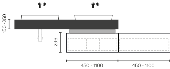
VL10 1 Ladenelement (Siphon-Lade) 1 Ladenelement (Standard-Lade)
