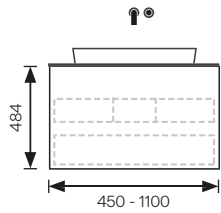
PLA01 1 Ladenelement (Standard-Lade und Siphon-Innenlade)*
