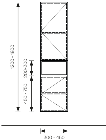
FI03 2 Drehtüren mit Anschlag rechts 4 Fächer innenliegend 1 Fach offen
