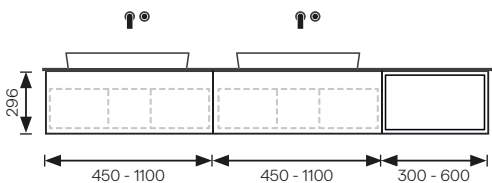
PLI08 2 Ladenelemente (Siphon-Laden)* 1 Offenes Element
