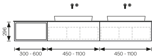
PLI07 1 Offenes Element 2 Ladenelemente (Siphon-Laden)*
