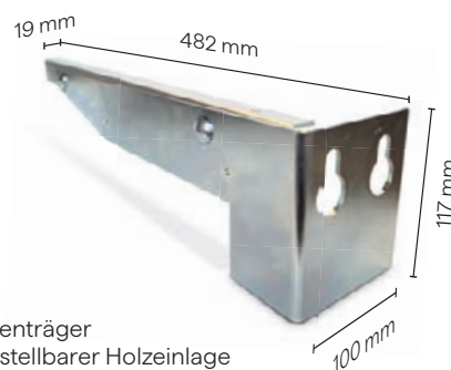
KT03 Konsolenträger mit Höhenausgleich
