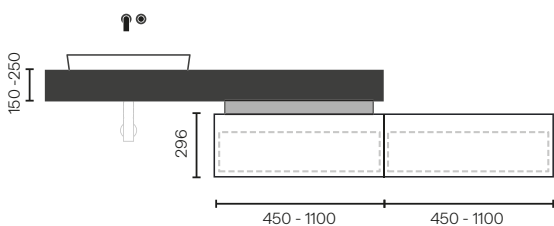
VL08 2 Ladenelemente (Standard-Laden)
